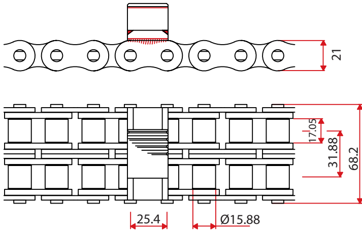
5218.000.10 Sharp top chain 16B-2
